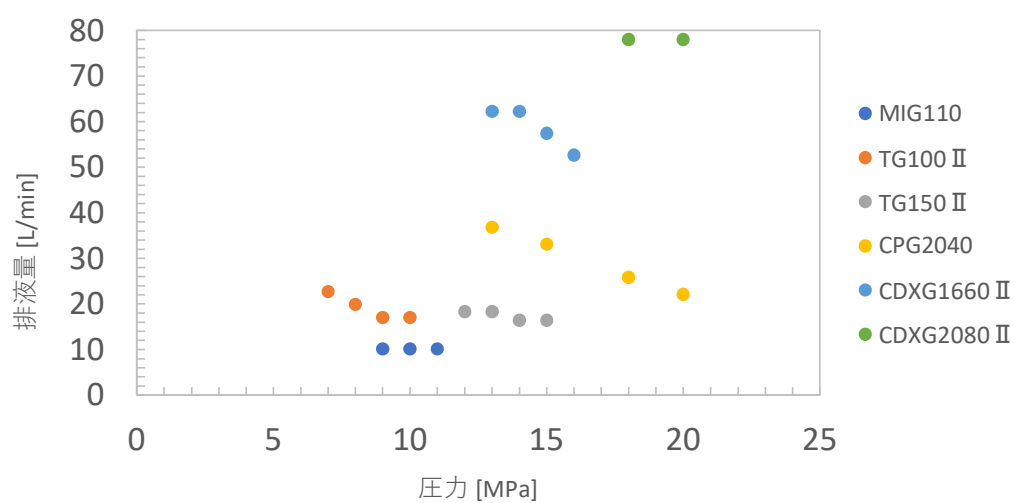
高圧洗浄シリーズ 性能曲線
