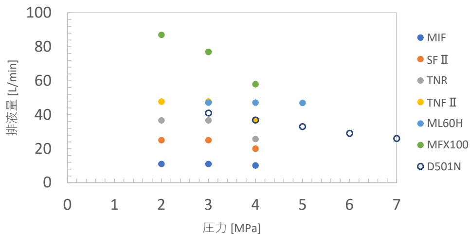
スタンダードタイプ 性能曲線
